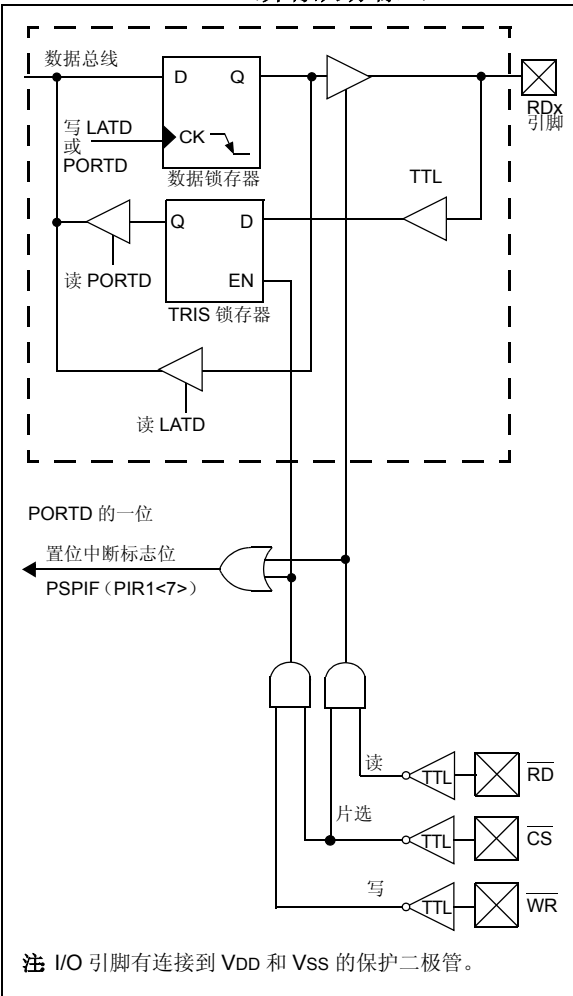
图 10-2: PORTD 和 PORTE 框图 (并行从动端口)
