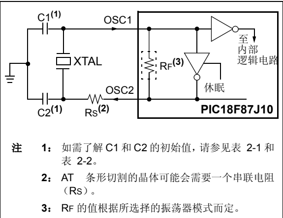
图 2-1：晶振 / 陶瓷谐振器的工作原理（HS 或 HSPLL 配置）
