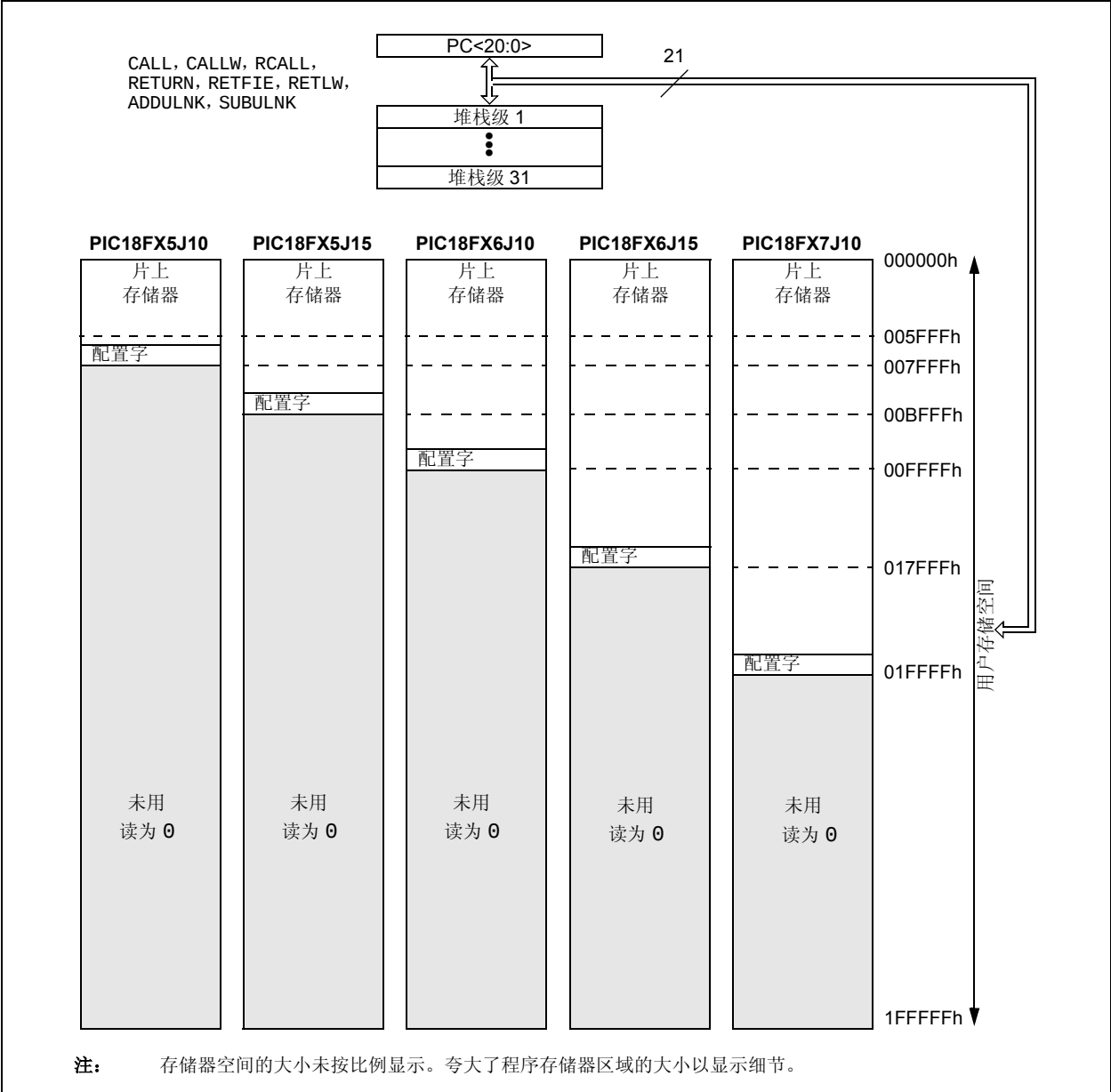
图 5-1: PIC18F87J10 系列器件的存储器映射图
