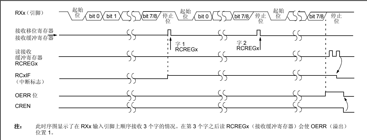
图 19-7: 异步接收
