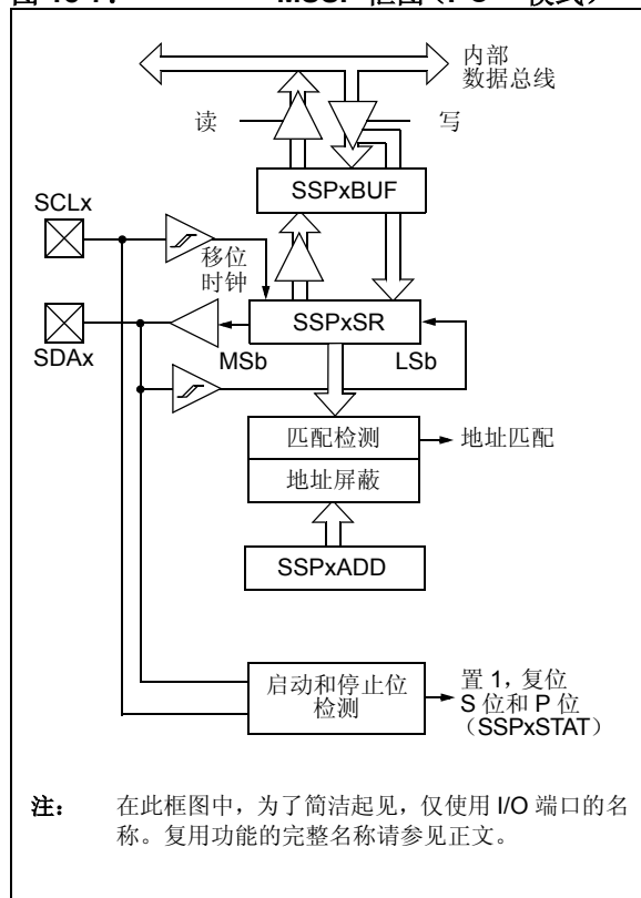
图 18-7: MSSP 框图 (I 2 C™ 模式)
