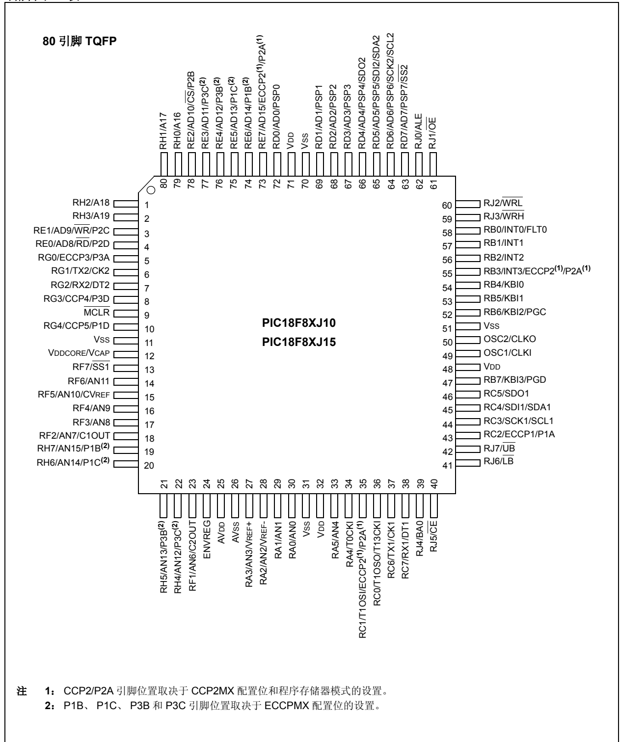
引脚图 (续)
