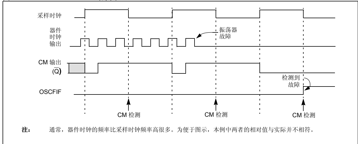
图 23-5: FSCM 时序图
