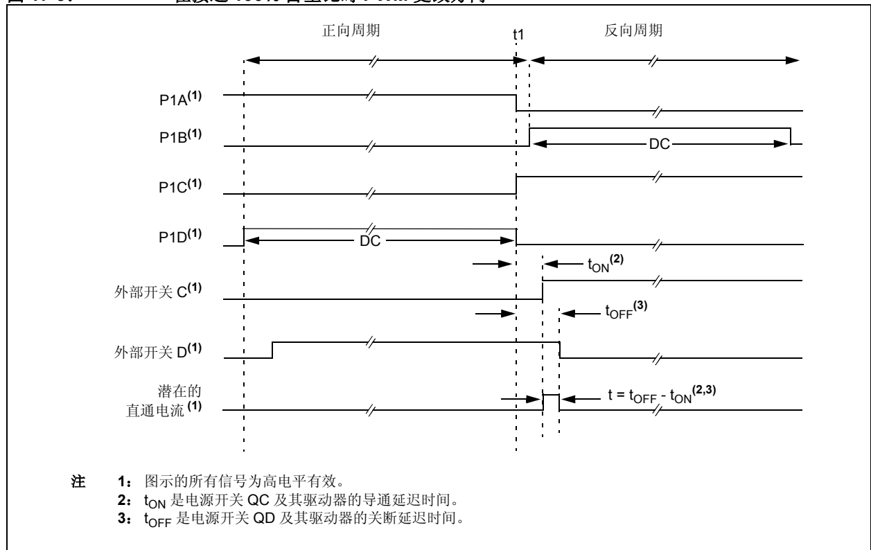
图 17-9: 在接近 100% 占空比时 PWM 更改方向
