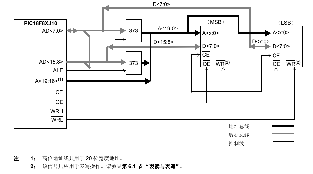
图 7-1: 16 位字节写模式示例
