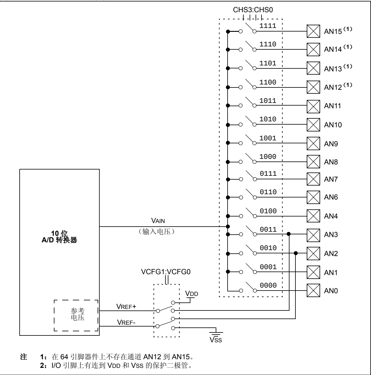
图 20-1: A/D 的框图
