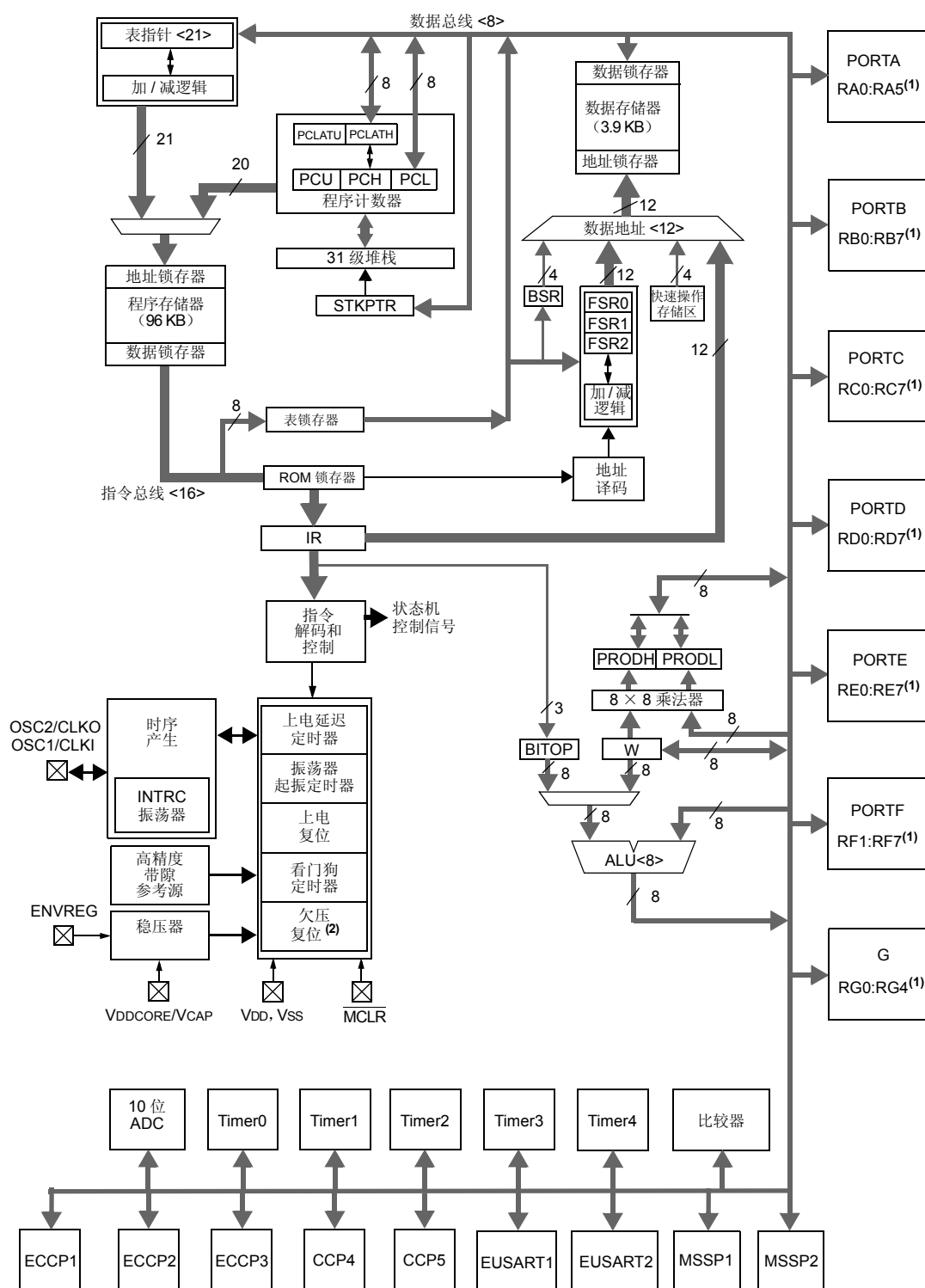
图 1-1: PIC18F6XJ10/6XJ15 (64 引脚) 框图
