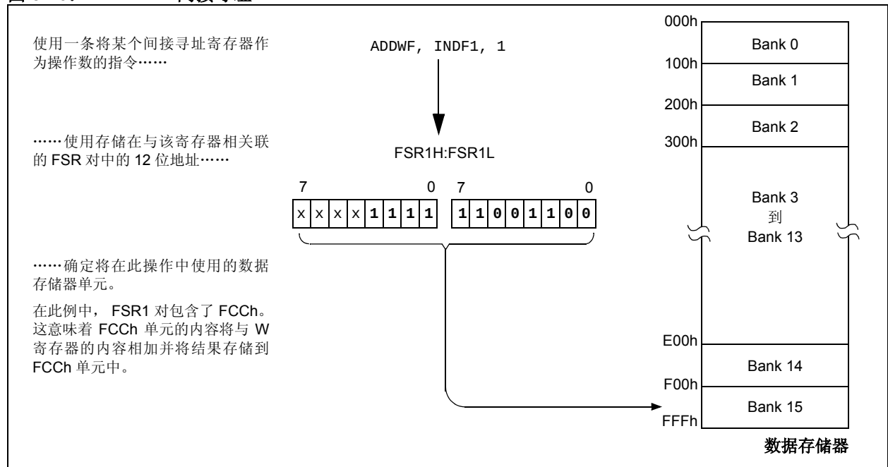
图 5-10: 间接寻址
