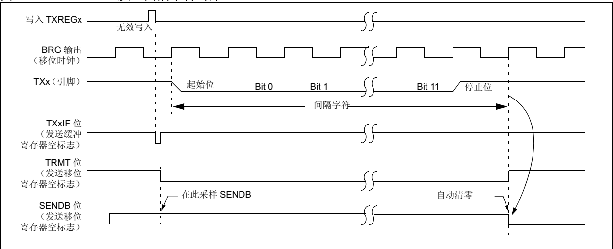
图 19-10: 发送间隔字符时序
