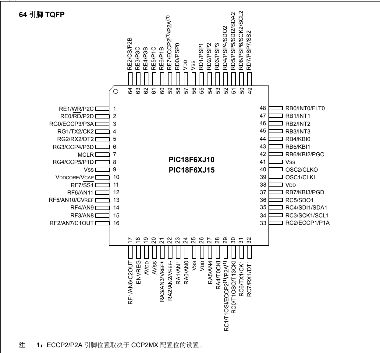
引脚图
