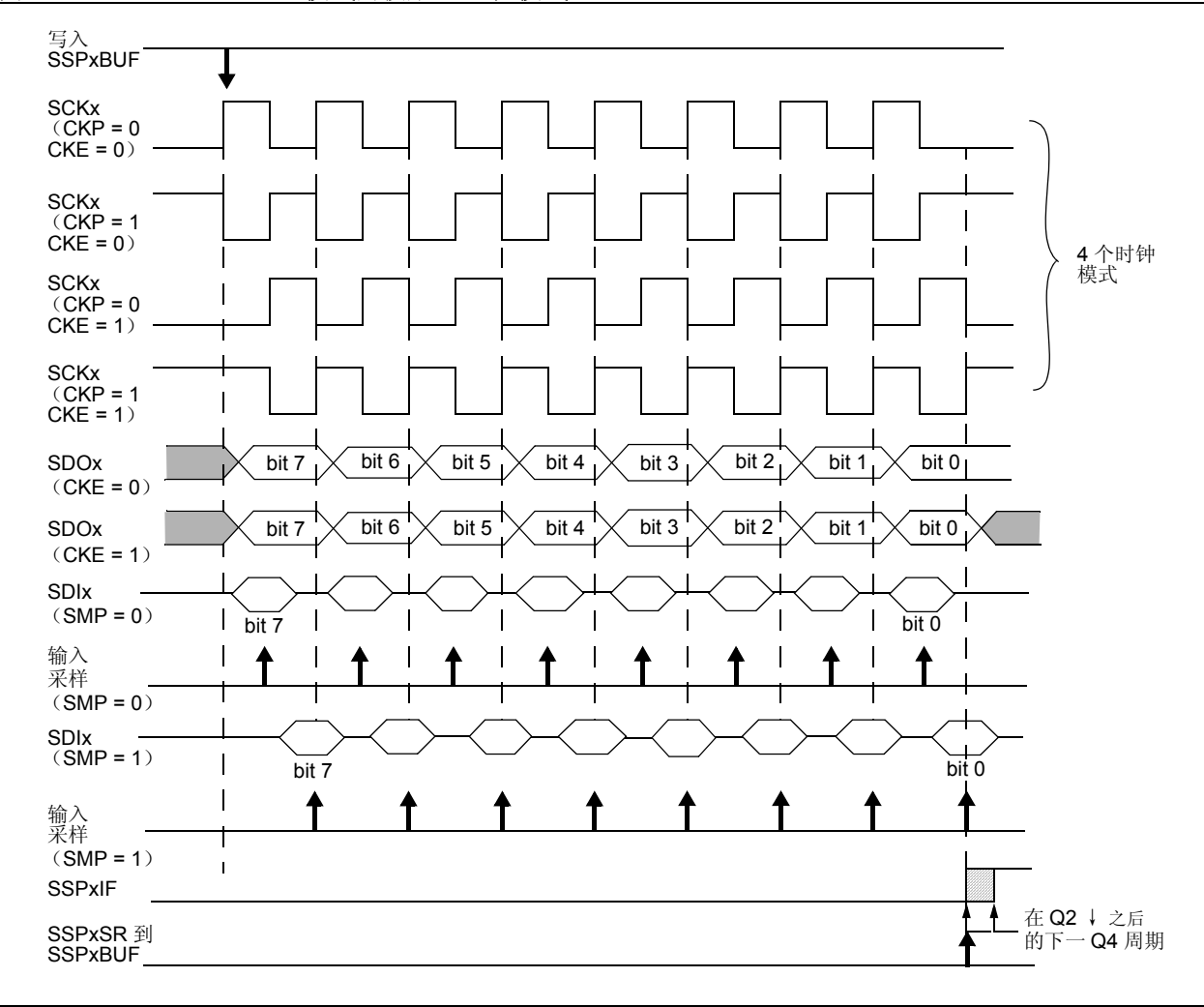
图 18-3: SPI™ 模式的波形（主控模式）
