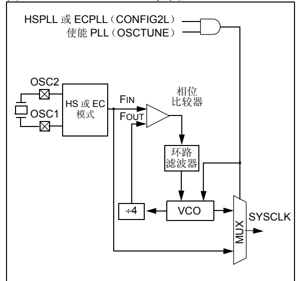
图 2-4: PLL 框图
