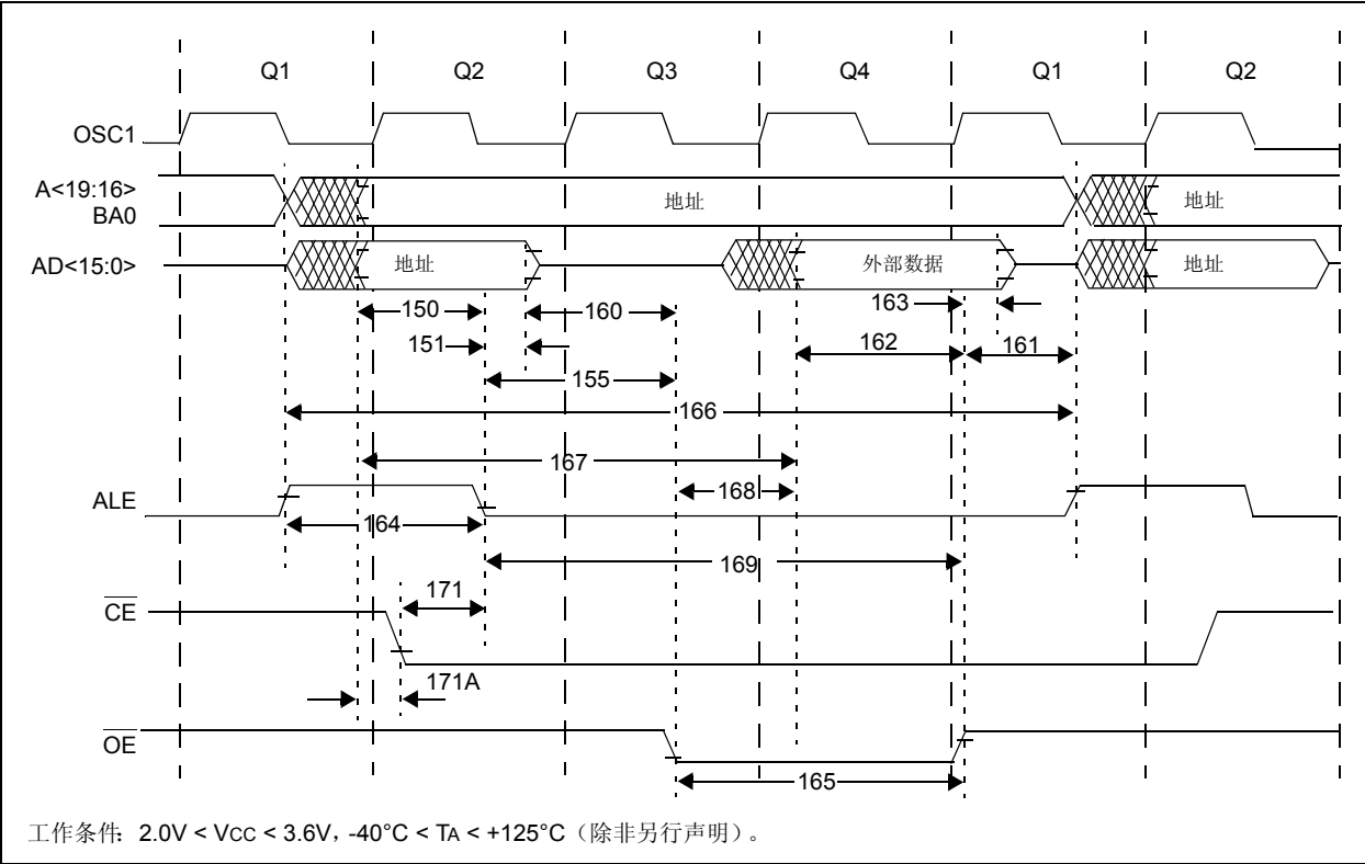
图 26-5: 读程序存储器时序图
