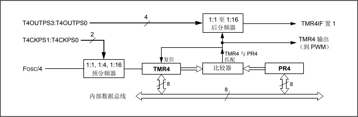
图 15-1: TIMER4 框图
