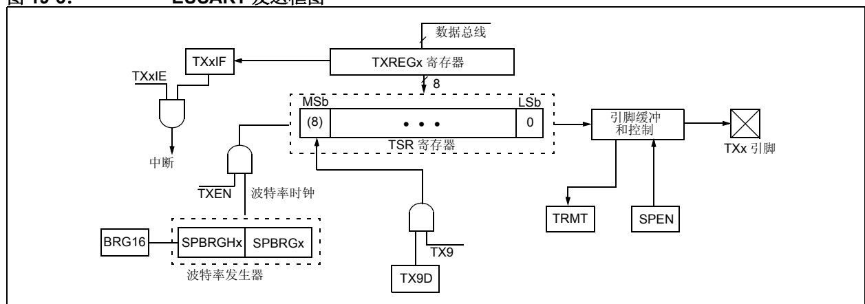
图 19-3: EUSART 发送框图
