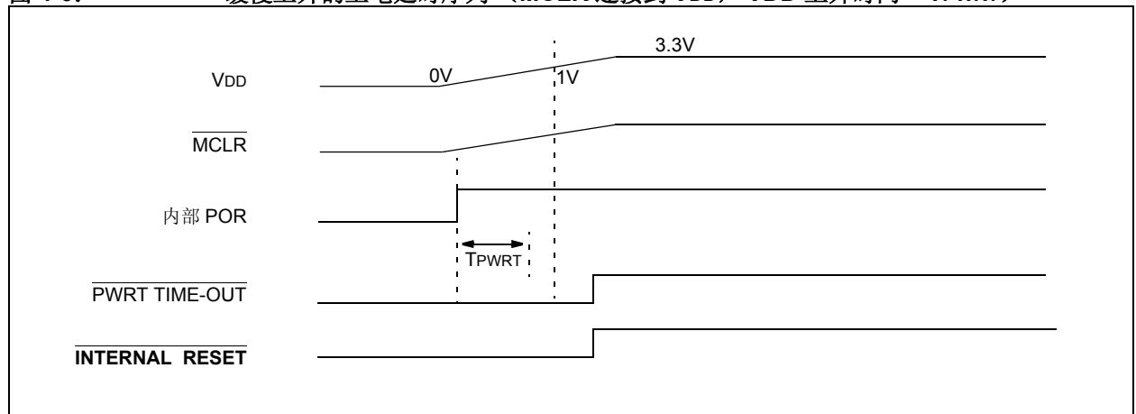
图 4-6: 缓慢上升的上电延时序列 ( \overline{\text{MCLR}} 连接到 \text{VDD} , \text{VDD} 上升时间 > \text{TPWRT} )
