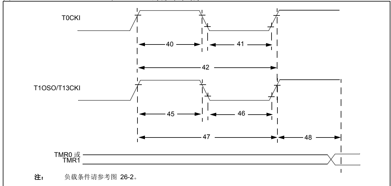
图 26-8: TIMER0 和 TIMER1 外部时钟时序
