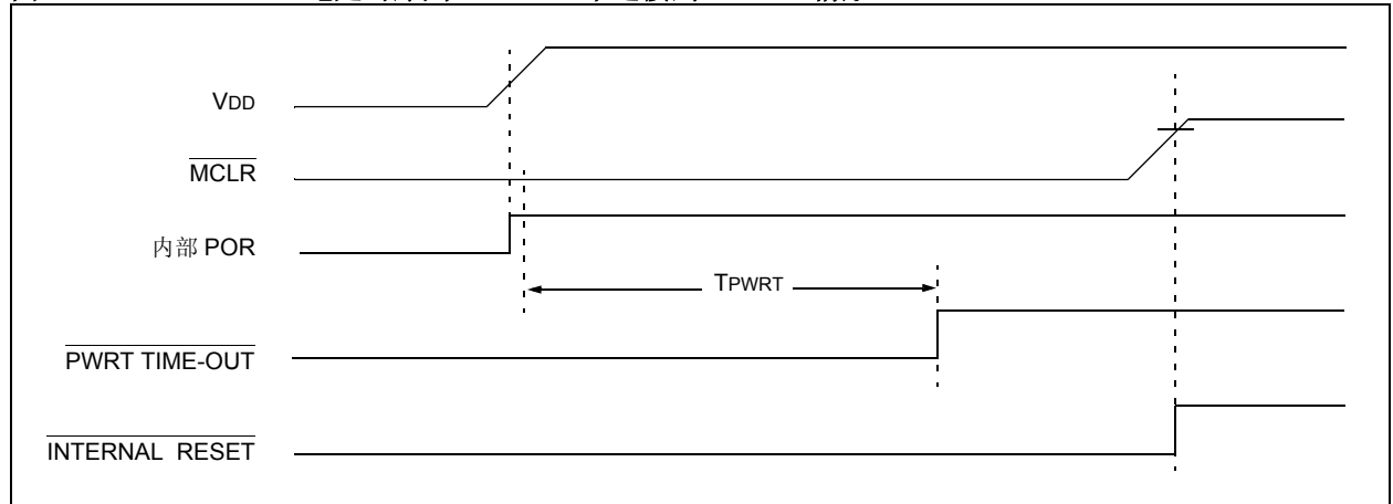
图 4-5: 上电延时序列 ( \overline{\text{MCLR}} 未连接到 \text{VDD} ): 情形 2
