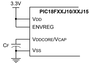
图 23-2: 片内稳压器连接
