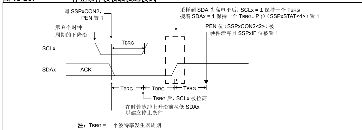
图 18-26: 停止条件接收或发送模式
