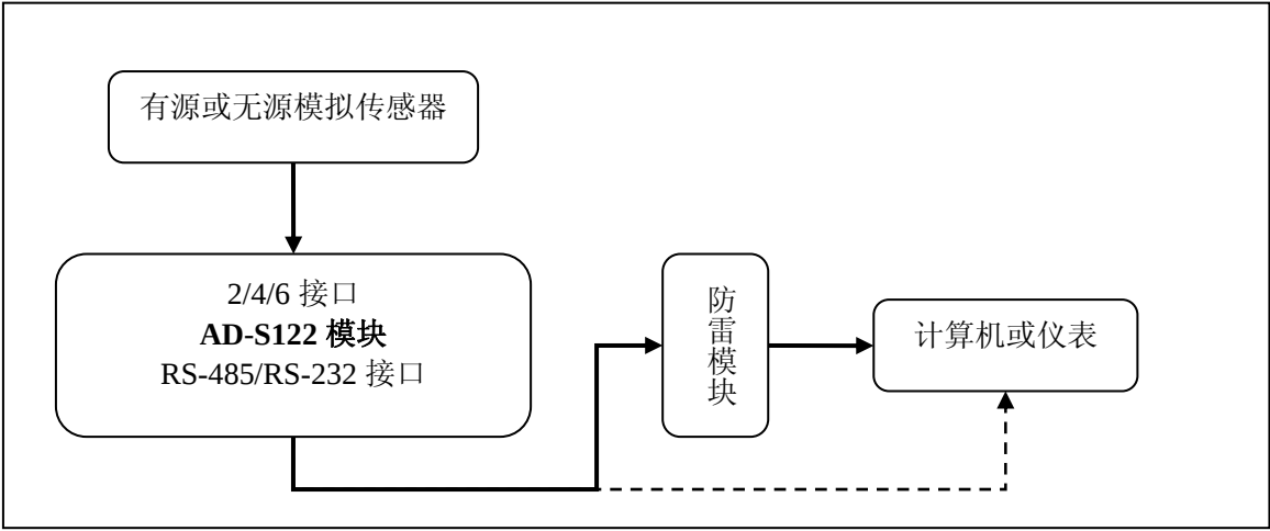
图 3-1 AD-S122 模块与传感器及仪表或计算机连接图
