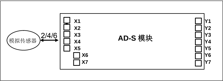
图 3-2 AD-S122 模块与传感器的连接图
