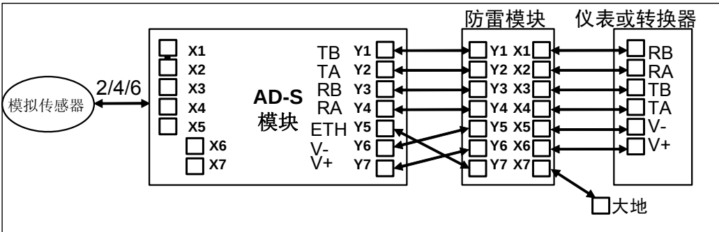
图 3-3 含有防雷板的仪表连接图
