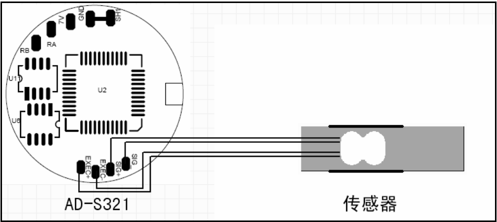
图 7-1 AD-S321 模块与传感器的连接图
