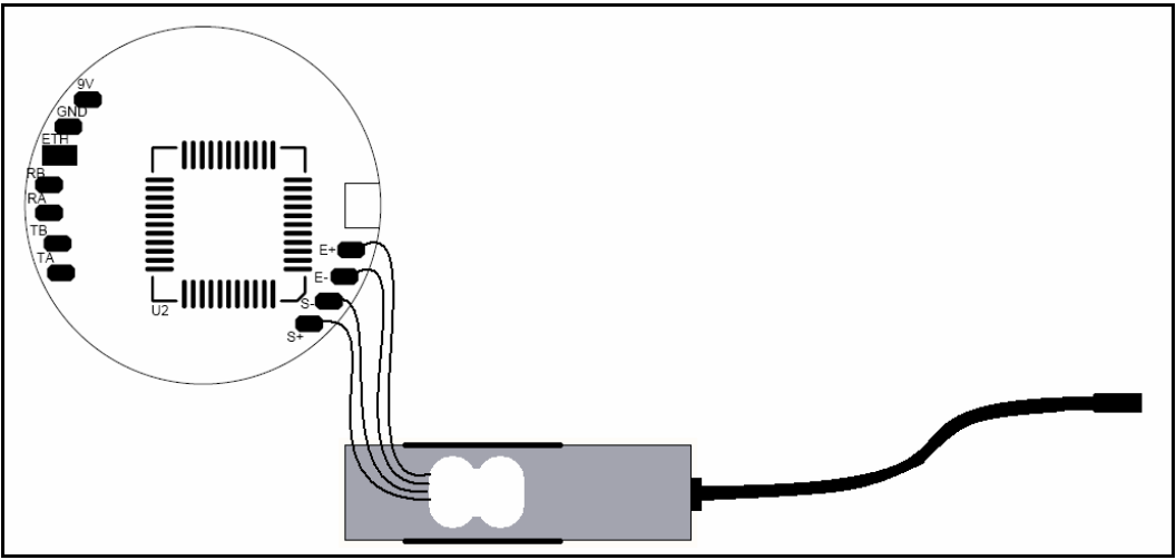
图 8-1 AD-S322 模块与传感器的连接图
