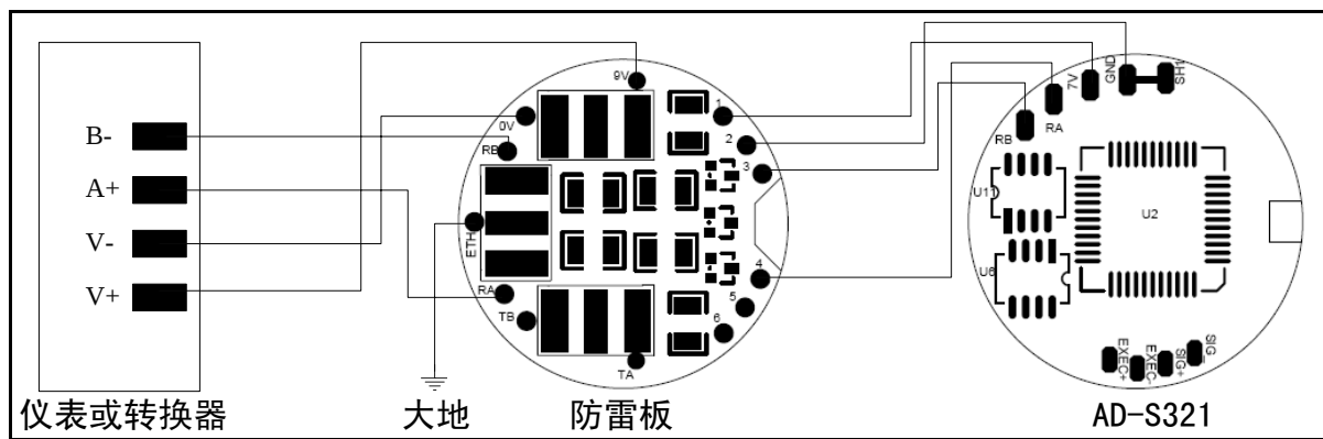
图 7-3 AD-S321 与防雷板相连的连接图
