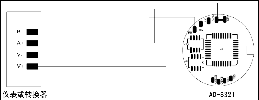
图 7-2 AD-S321 直接与仪表相连的连接图
