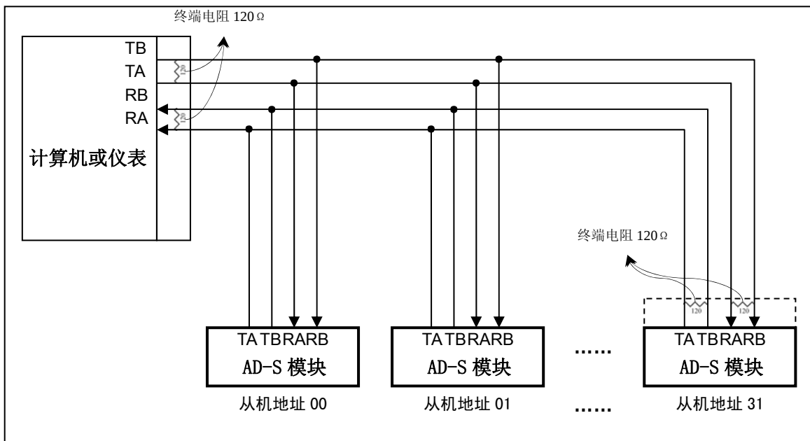
图 3-5 AD-S122 模块的总线结构图
