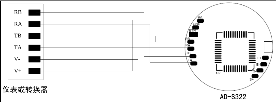
图 8-2 AD-S322 直接与仪表相连的连接图
