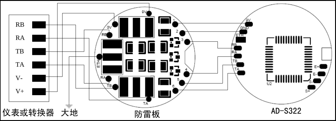
图 8-3 AD-S322 与防雷板相连的连接图
