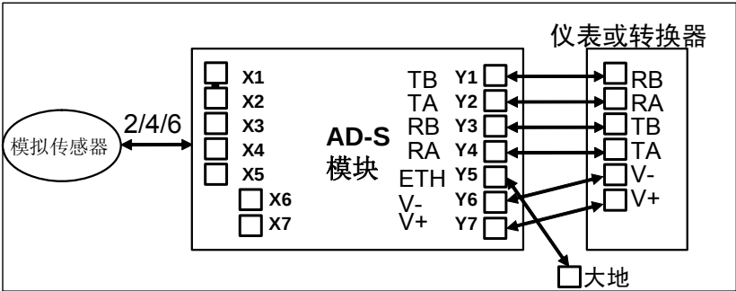
图 3-4 AD-S122 直接与仪表相连的连接图
