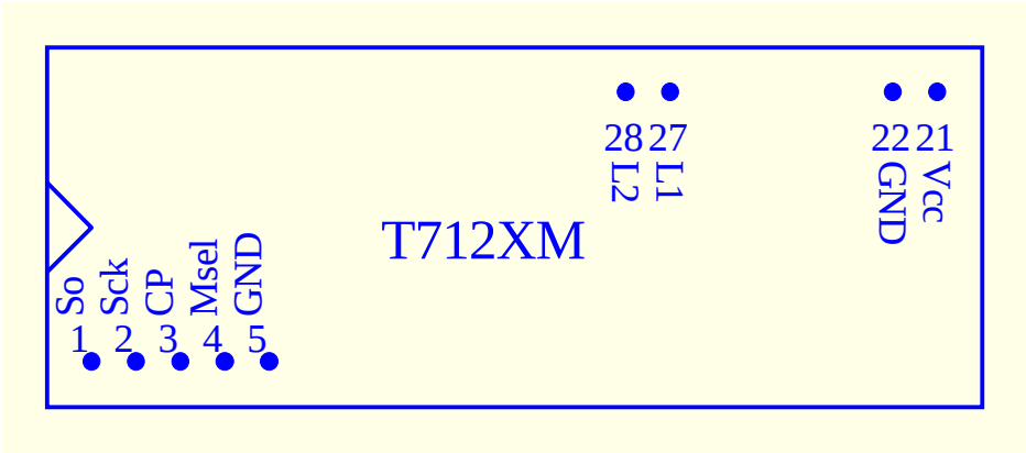
顶 视 图
